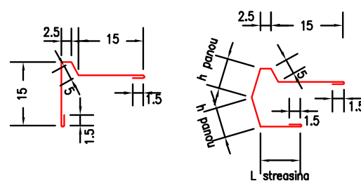
12. Bordură de fronton
