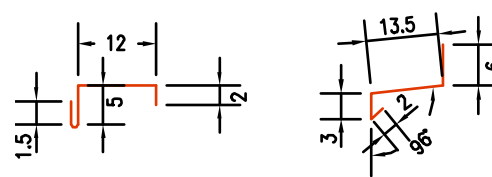
14. Șorț de soclu
