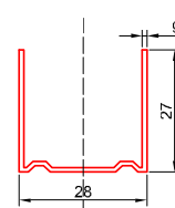
16. UW28
