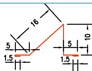
6. Parazăpadă
