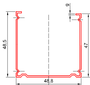
21. CW50
