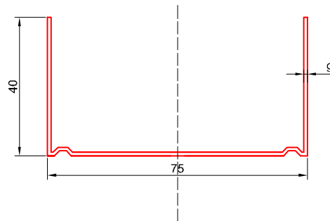
18. UW75
