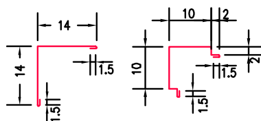
13. Bordură de colț
