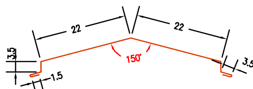
4. Coamă cu panta dublă
