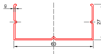
20. CD60
