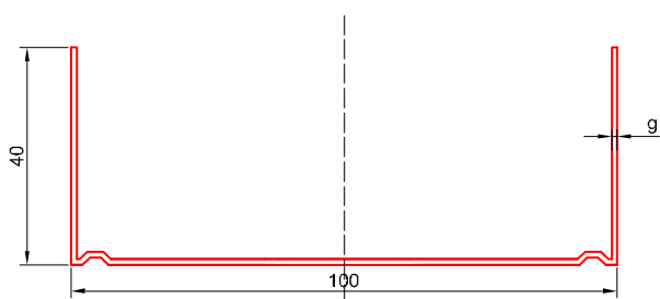
19. UW100
