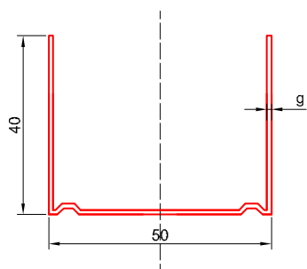
17. UW50
