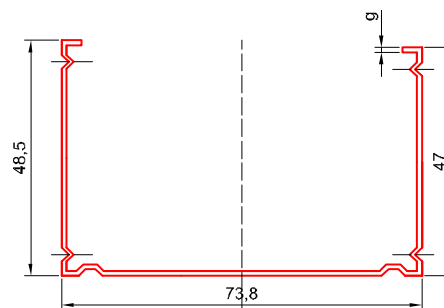
22. CW75
